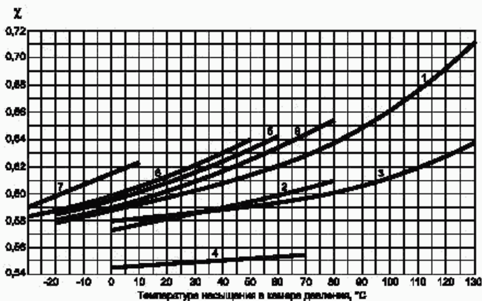
Рисунок Б.3 — Значение коэффициента \chi для критического давления потока.
